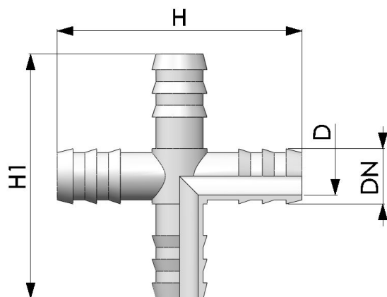
PORTAGOMMA CROCE per tubo DN
